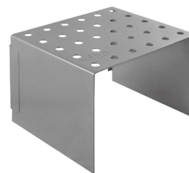
59813 4 SF 30孔起子架 適用於所有雙色柄系列
