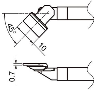
T51-LA10 / SOP 10LA 型
