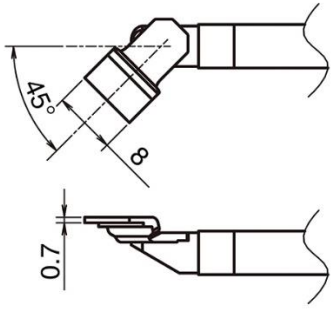
T51-LA8 / SOP 8LA 型
